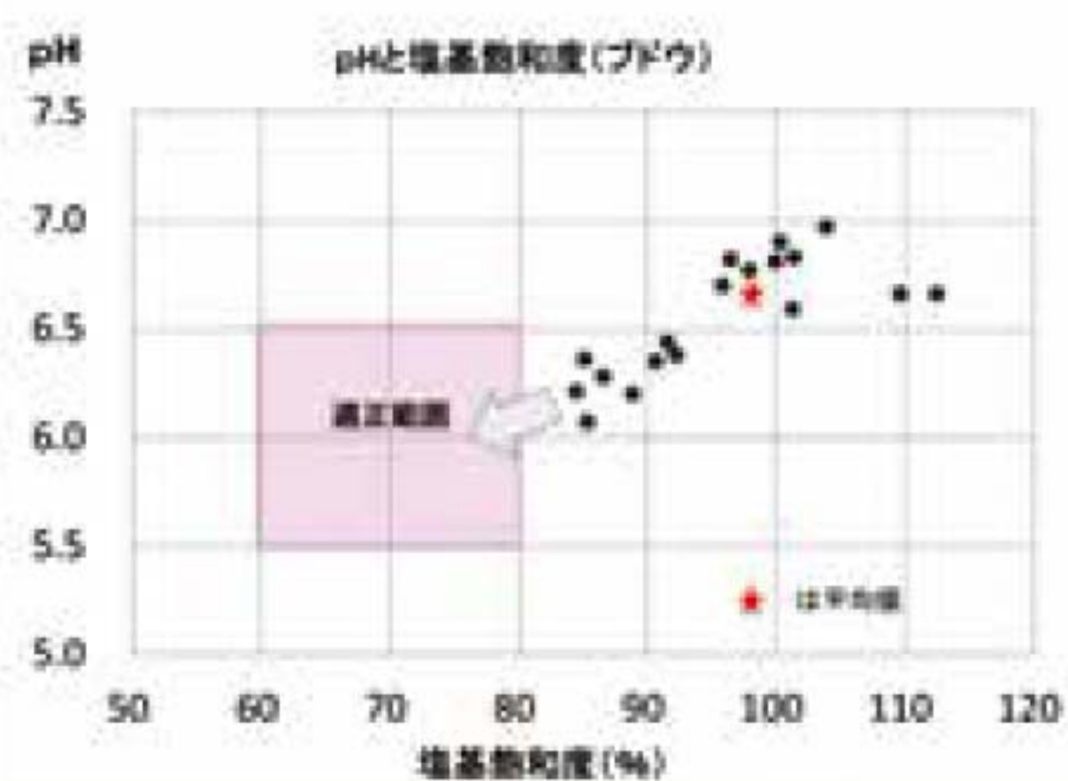
図1 pHと塩基飽和度 (ブドウ)
