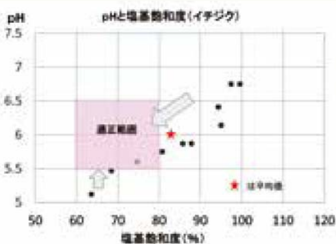
図2 pHと塩基飽和度 (イチジク)
